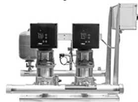
2017 ComBo HP Druckerhöhungs- anlagen
